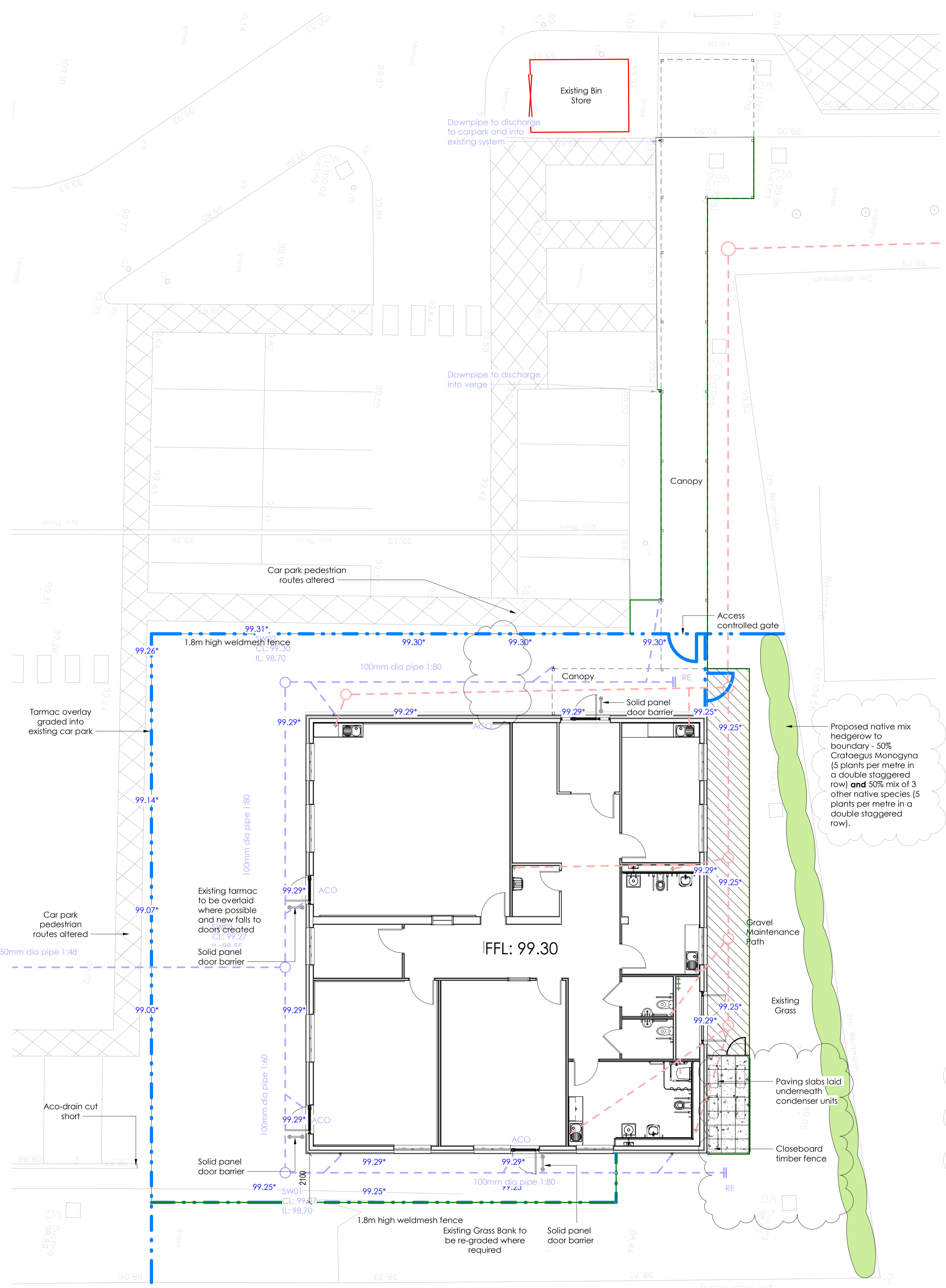
Landscaping Plan 1 : 100
