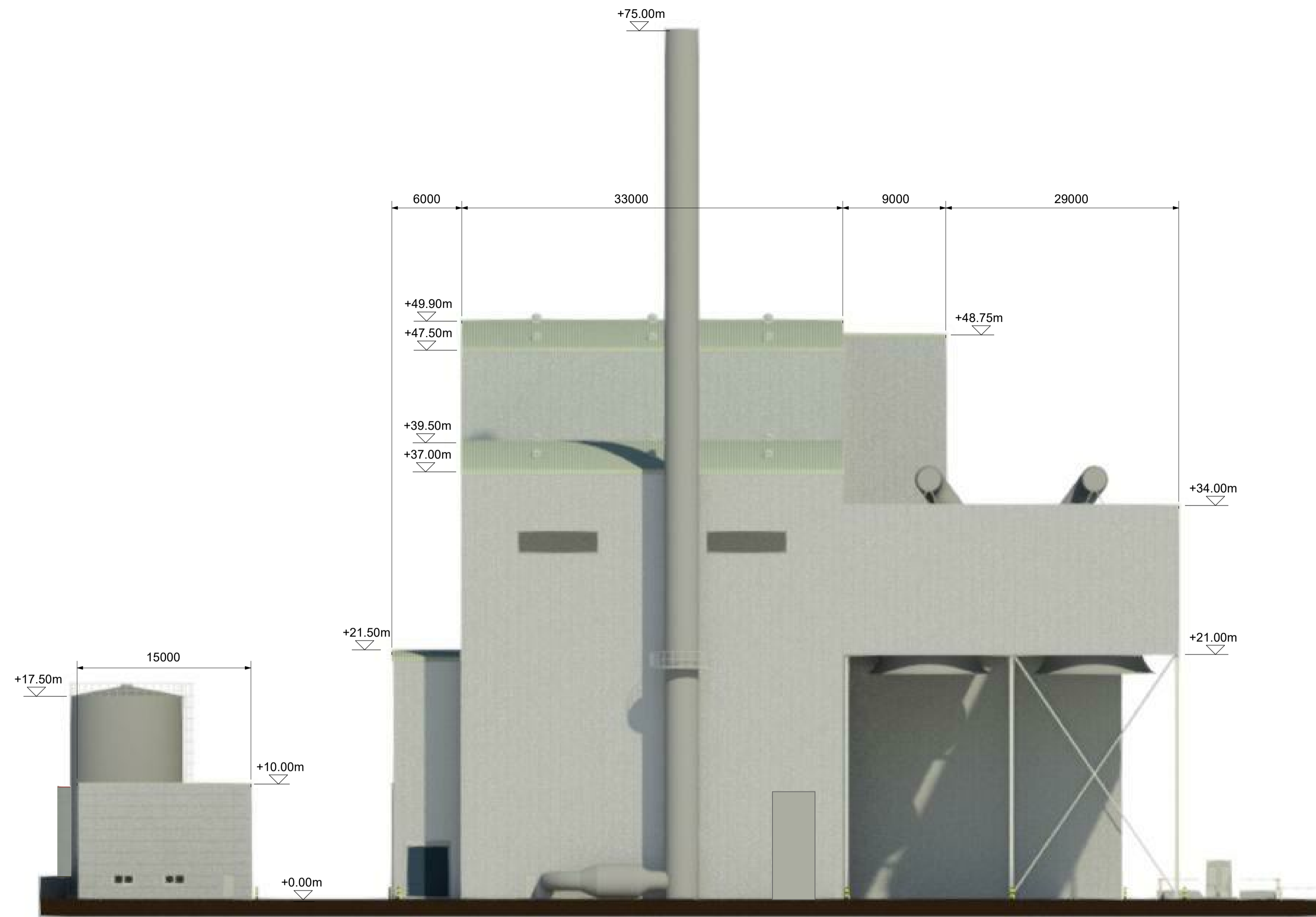
D West Elevation 1:1 NTS
